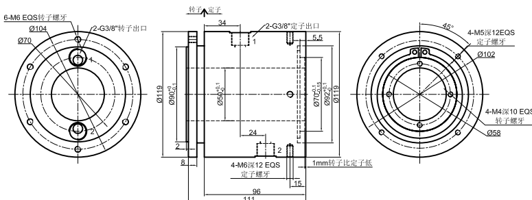
GJ2050-04 外形尺寸图
