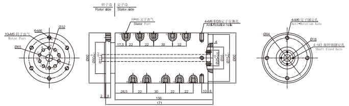
▼ MAPH1000-01气电一体 尺寸图
